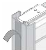
Ⓐ1 U-list med tejp och vinkel. Till modell 3242 levereras vinkel tillsammans med wirefoot. Sidolisten kan också monteras på glas.
