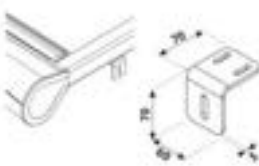
L-monteringsvinkel nischmontage 70x70 mm
