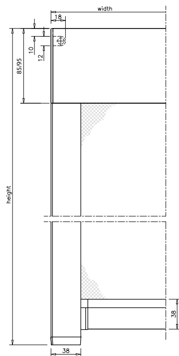
Kassett, sido- och underlist – motorutgång baktill
