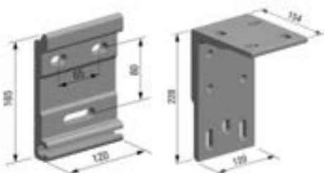
Standardbeslag tak/vägg
