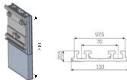
Lodrät monteringsplatta för vägg inkl. standardbeslag
