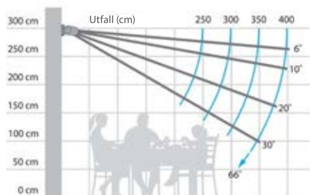
Montering vägg
