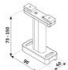
Monteringsbeslag sidoskenor. Höjd 150 mm, kan kortas av till 73 mm. 120 mm är minsta höjd vid minst 4x4 m markis.
