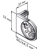
Sidobeslag, Design Standard
