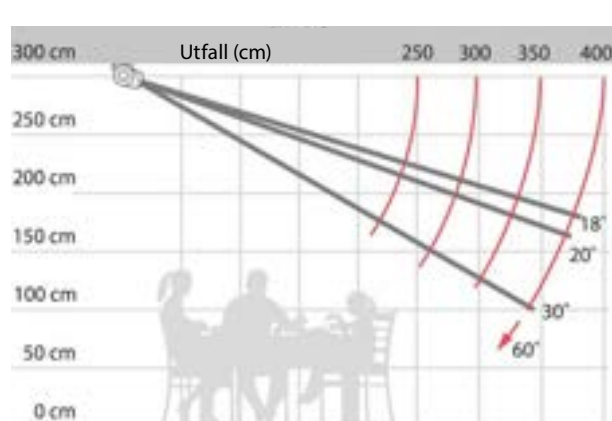
Montering tak
