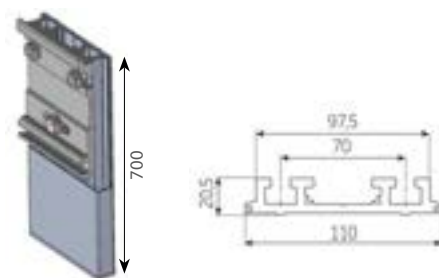
Lodrät monteringsplatta för vägg inkl. standardbeslag Se sid 33 för ytterligare info om montering.
