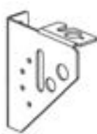
Nischfäste Fem olika djup: 45, 65, 100, 130 och 185 mm.
