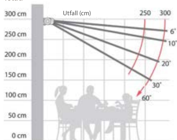
Montering vägg
