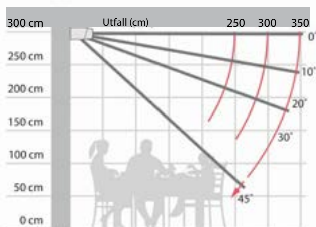
Montering tak
