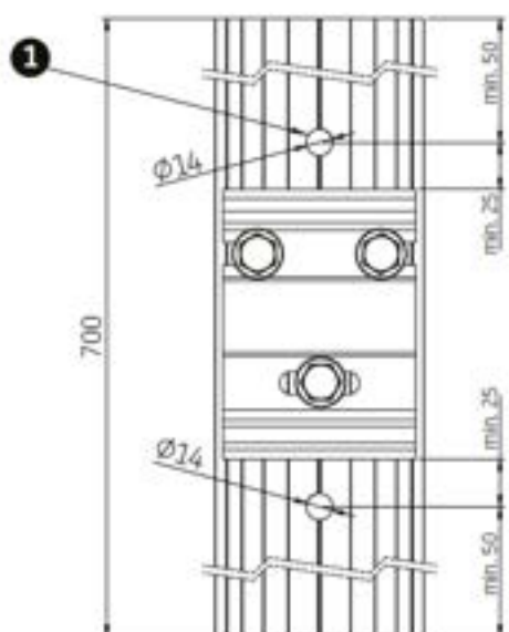
Minsta avstånd mellan infästning och väggbeslag/ ytterkant monteringsplatta
