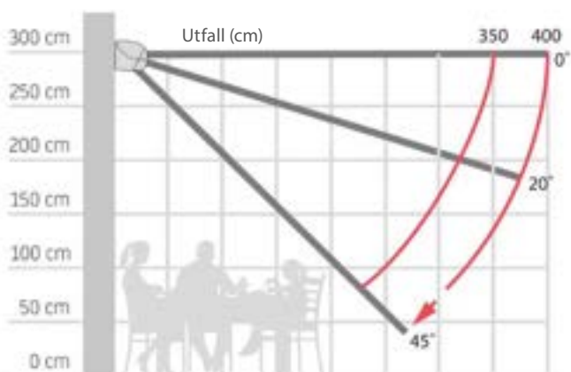
Montering vägg
