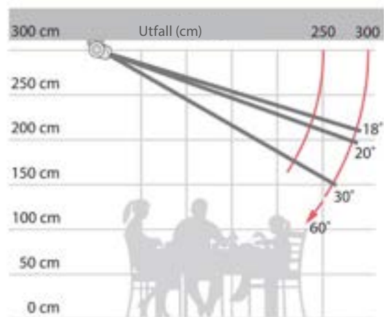
Montering tak
