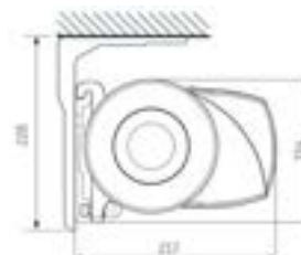
Takmontering med L-vinkel
