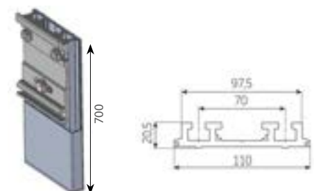
Lodrät monteringsplatta för vägg inkl. standardbeslag
