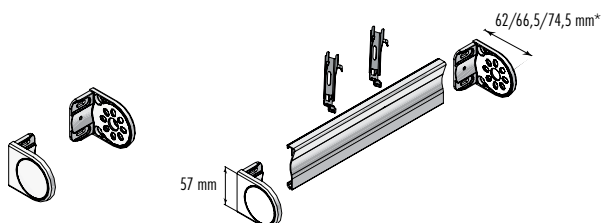
Modell 10 Sidobeslag
