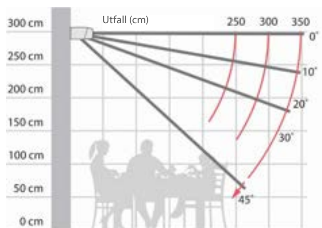
Montering vägg
