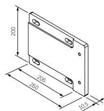
Monteringsplatta för tak. Takbeslaget skruvas fast i takplattan
