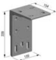
L-vinkel för tak (standardbeslag medföljer)
