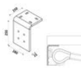
L-vinkel för tak kombineras med väggbeslag
