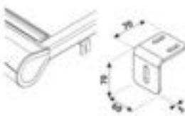
L-monteringsvinkel nischmontage 70x70 mm
