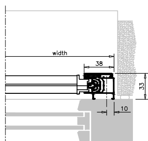
Tvådelad sidolist
