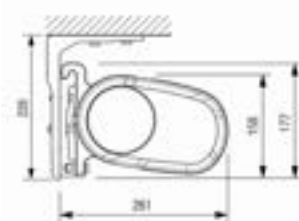
Takmontering med L-vinkel
