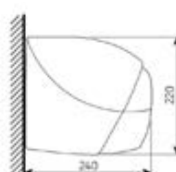
Bergen Kassett Väggmontering
