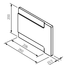
Stor monteringsplatta utan hål för tak eller vägg. Tak/Väggbeslaget skruvas fast i monteringsplattan
