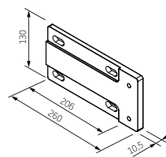
Smal monteringsplatta för vägg. Väggbeslaget skruvas fast i monteringsplattan
