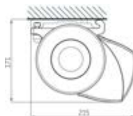
Takmontering
