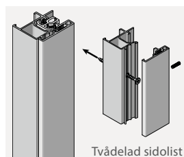
Tvådelad sidolist
